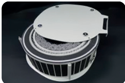
Vorfilterpaket, komplett
